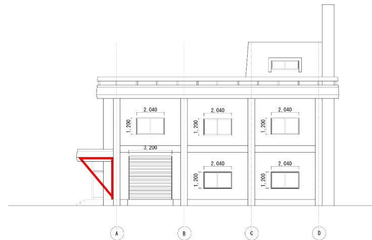
北側立面図（補強案）
