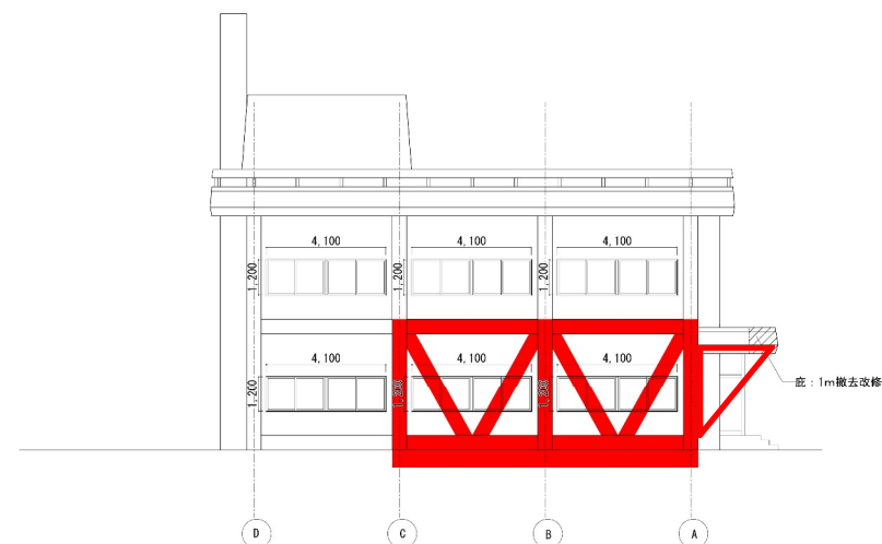
南側立面図（補強案）
