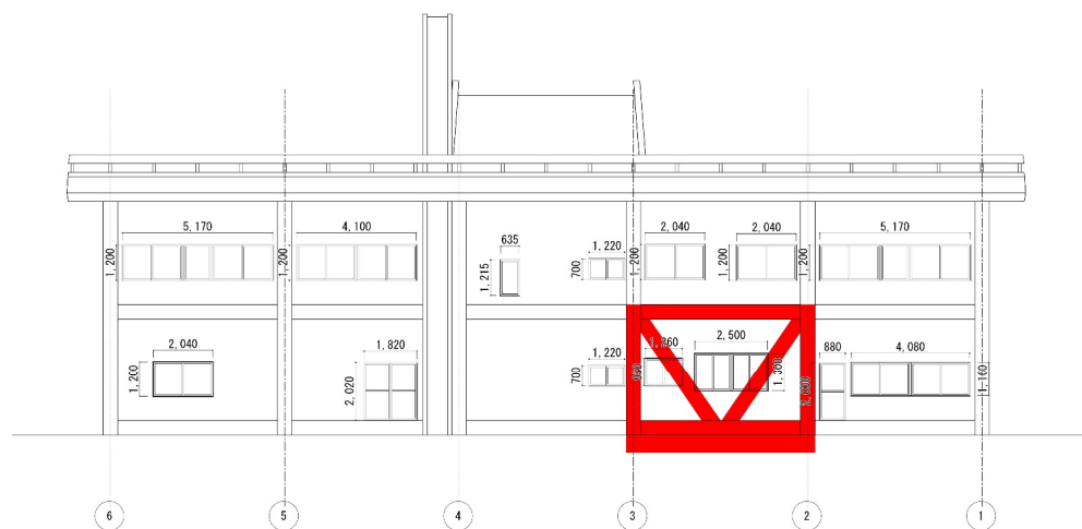
西側立面図（補強案）
