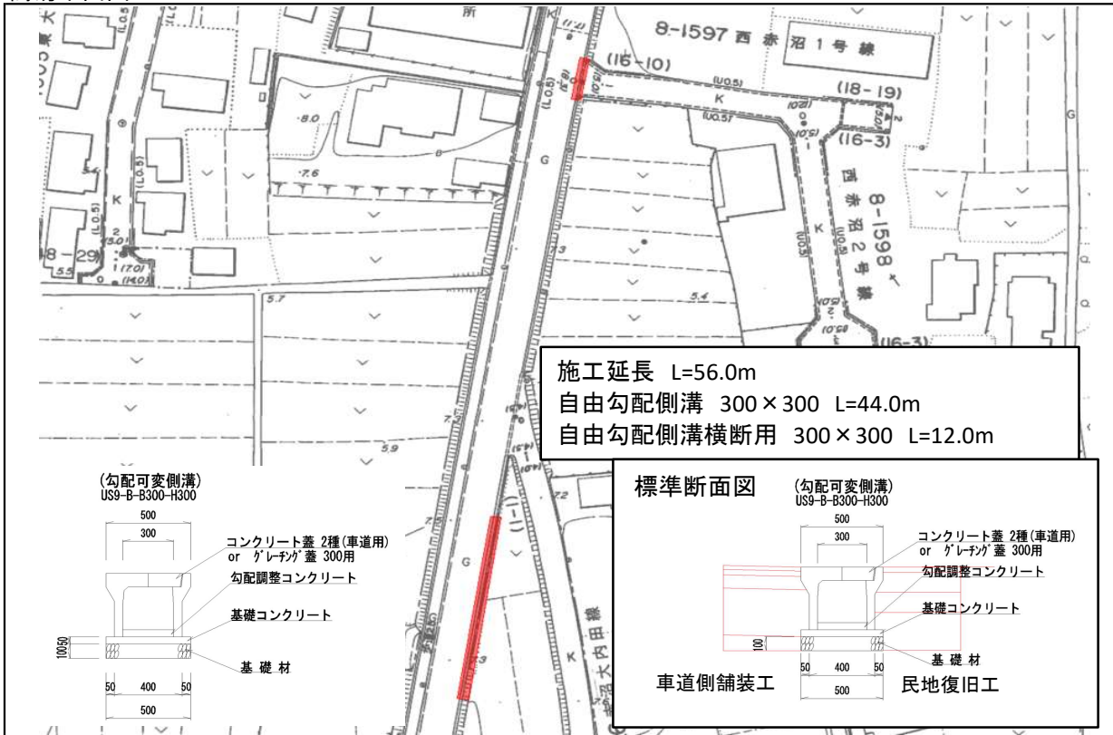
簡易平面図
