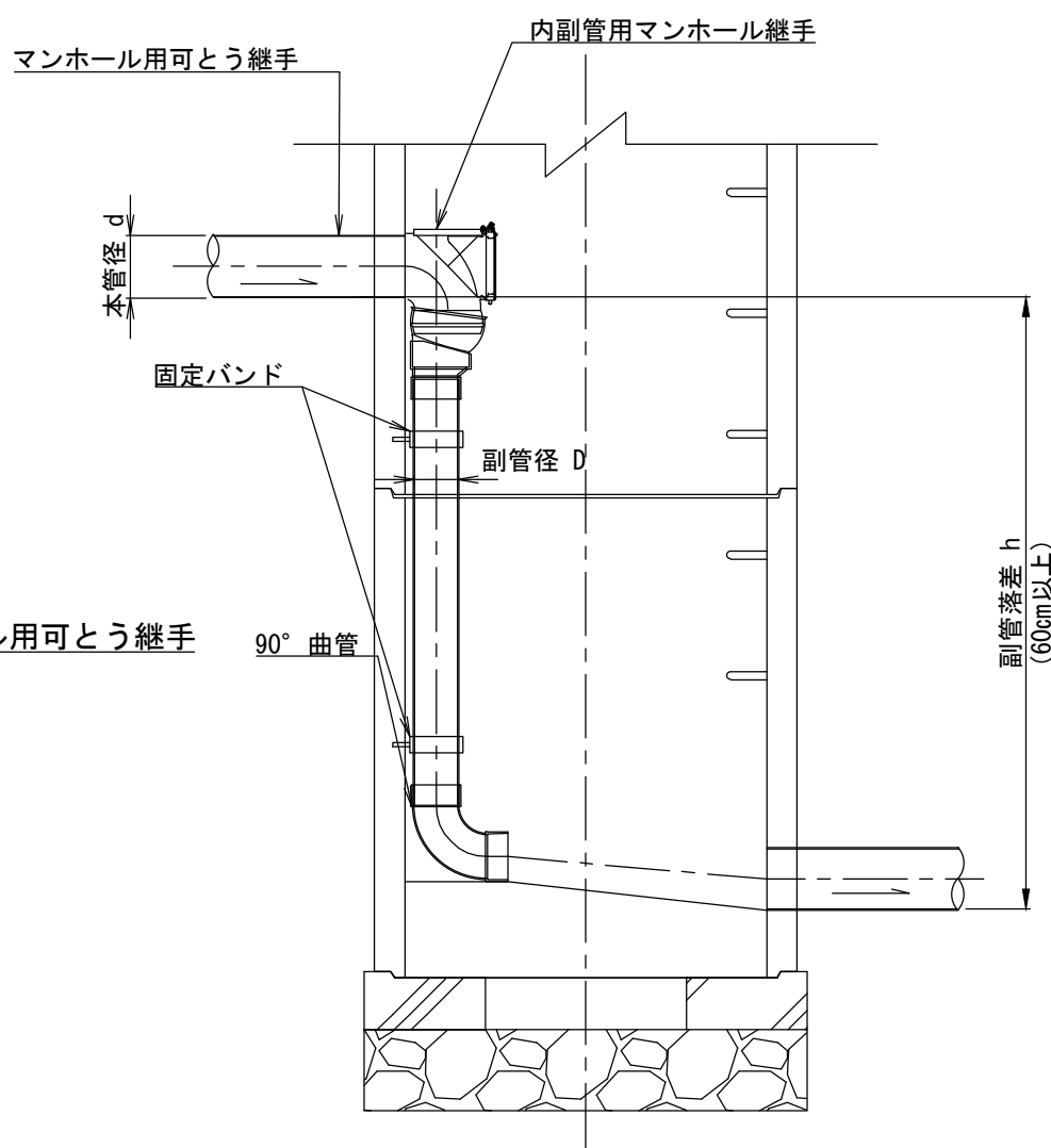
内副管寸法表(分流式)
