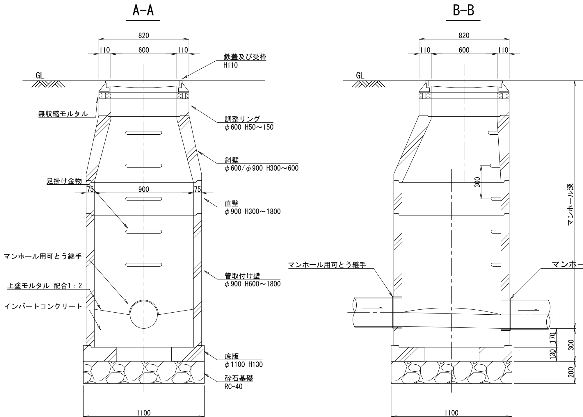
断面図
