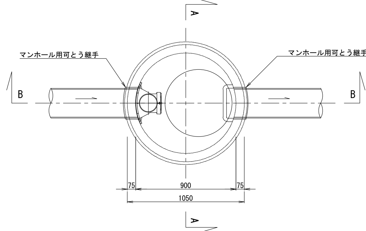
平面図
