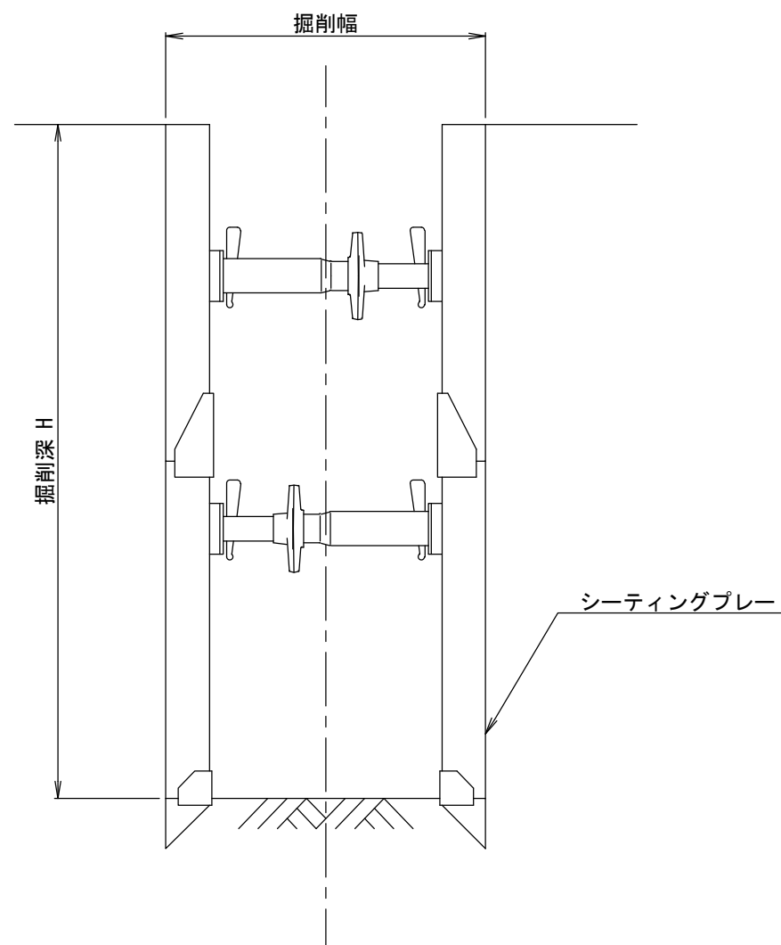
断面図
