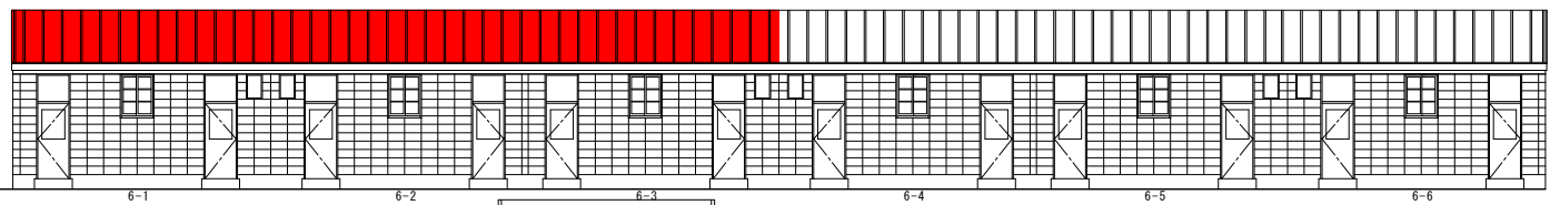
北立面図 S = 1 : 100
