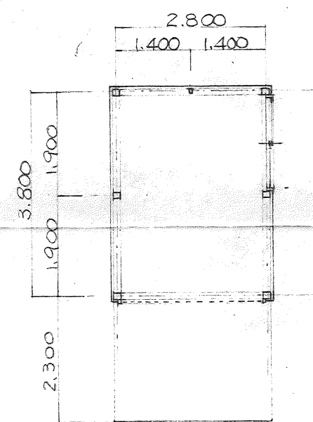
平面図 1/100 10.64㎡
