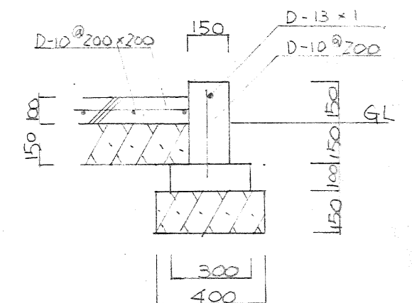
B 詳細図 1/20
