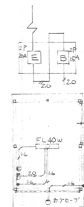
電気設備図 1/100
