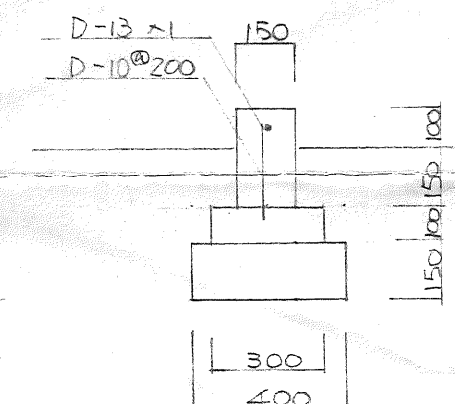
C 詳細図 1/20
