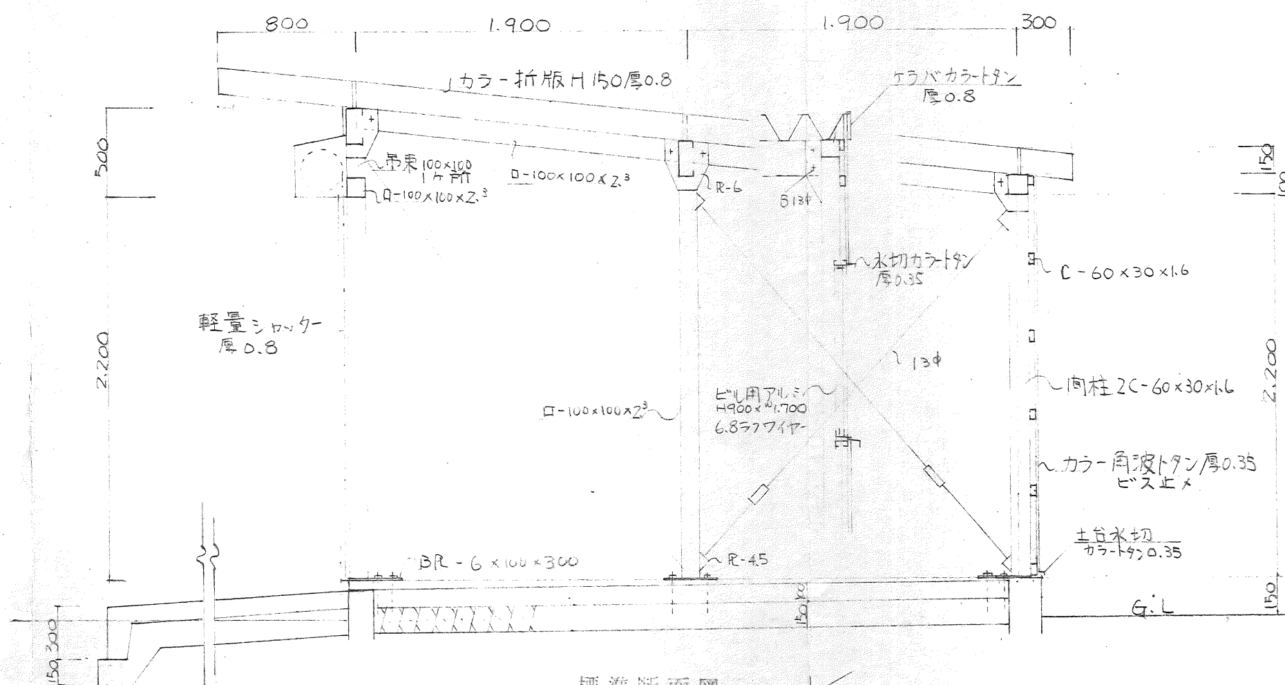
標準断面図 1/30
