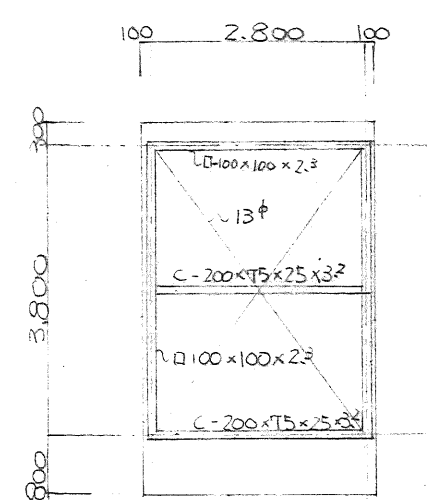
小屋伏図 1/100
