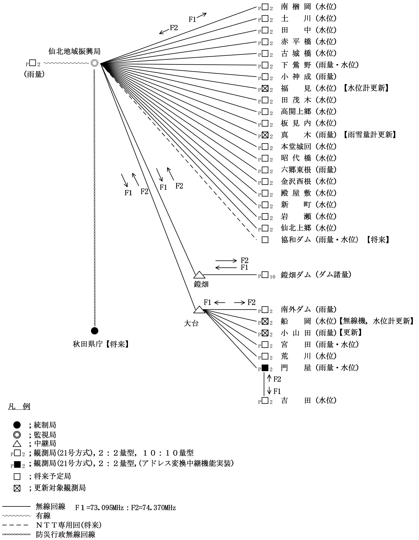
図2.1 回線構成図 (仙北)
